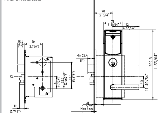
ANSI DA lockcase:
