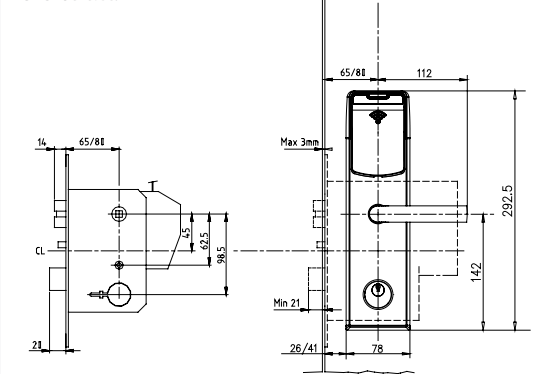
EURO lockcase:
